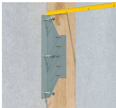
Instalace na min. vzdálenost
